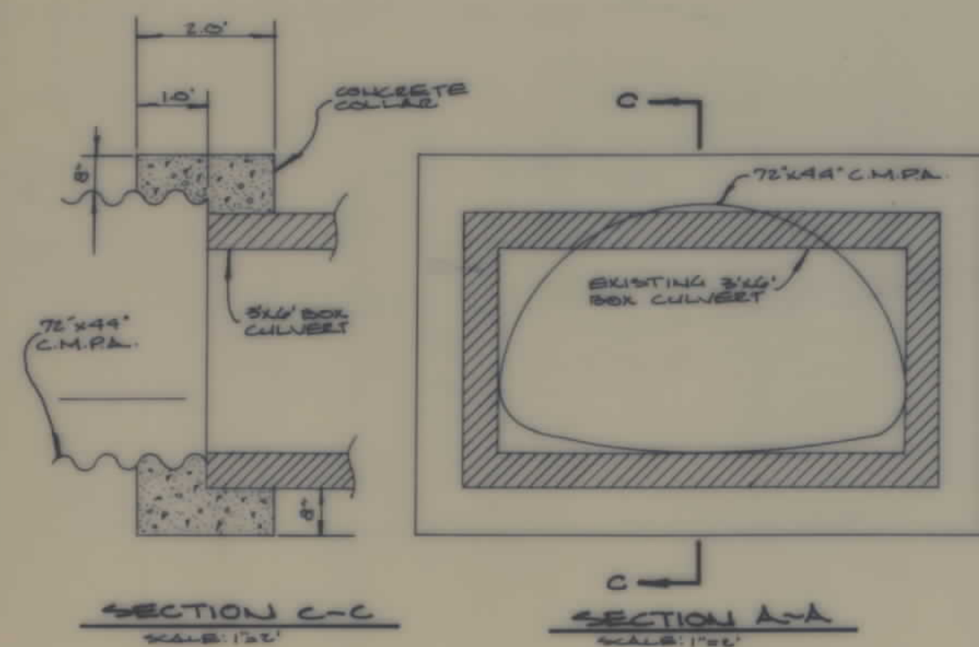
DETAIL STA. 27+00 CHEYENNE AVENUE SCALE: 1\"/>
