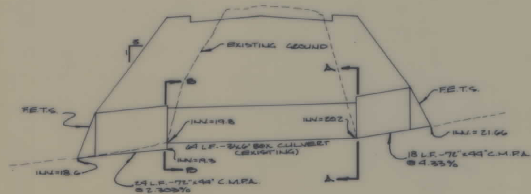
DETAIL STA. 27+00 CHEYENNE AVENUE SCALE: 1\"/>
